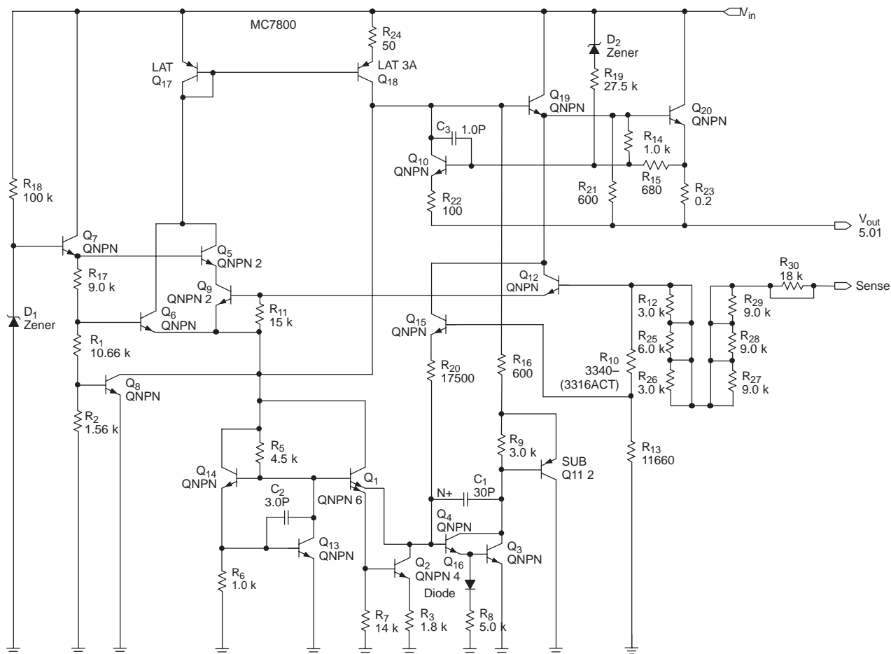
等価回路図
