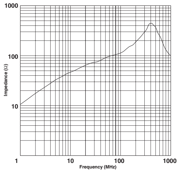
RRH080-032-101
