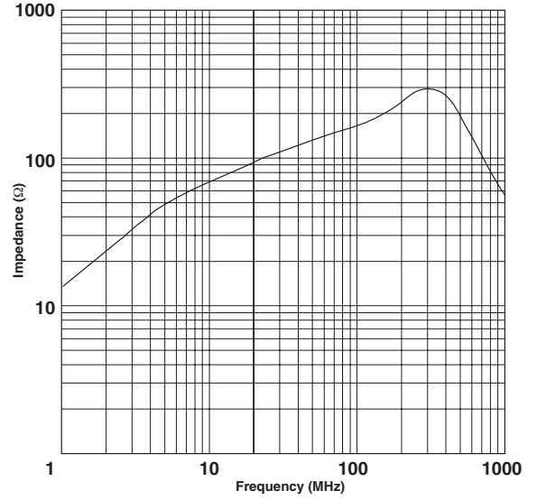
RRH190-058-315
