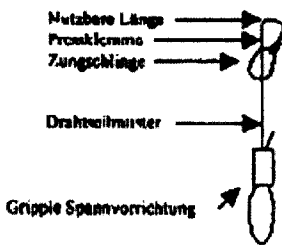
Mit Schlaufe
